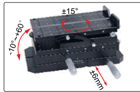
工作台(标配)
